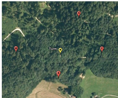
Endpunkte der 160m Dipole
